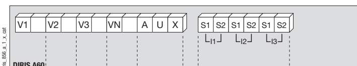
DIRIS A60
