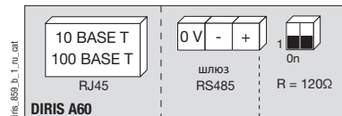
Модуль Ethernet + шлюз RS485 JBUS/MODBUS
